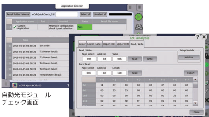
I2C解析画面
